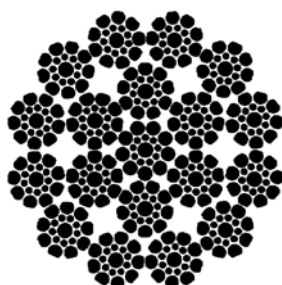
SFP 19 (19x19)
